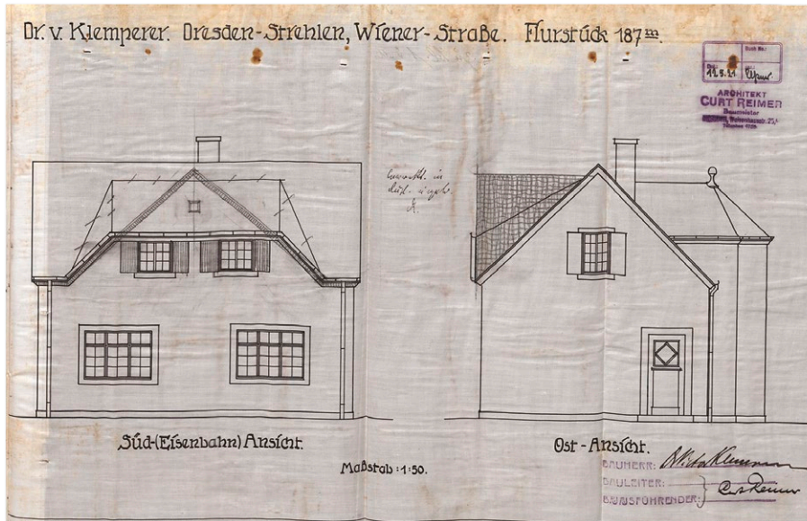
19 – Wiener Straße 126, Ansichten vom Wohnhaus, 1921
