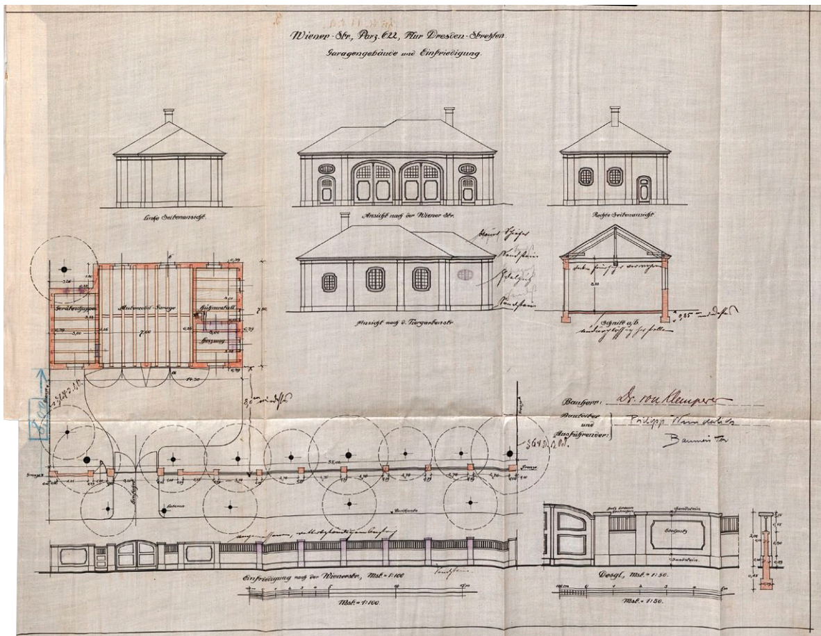
17 – Flurstück Nr. 622, Bauplan Garage, 1913
