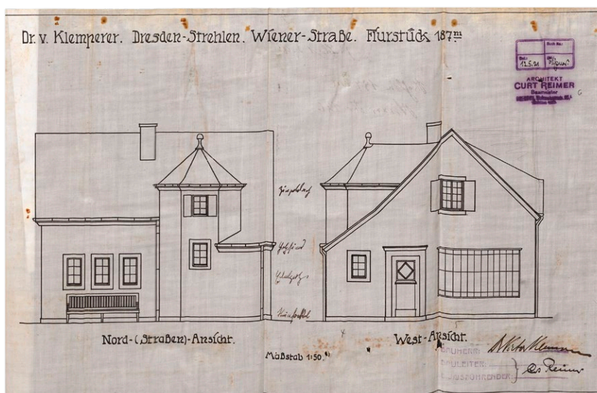
18 – Wiener Straße 126, Ansichten Wohnhaus, 1921
